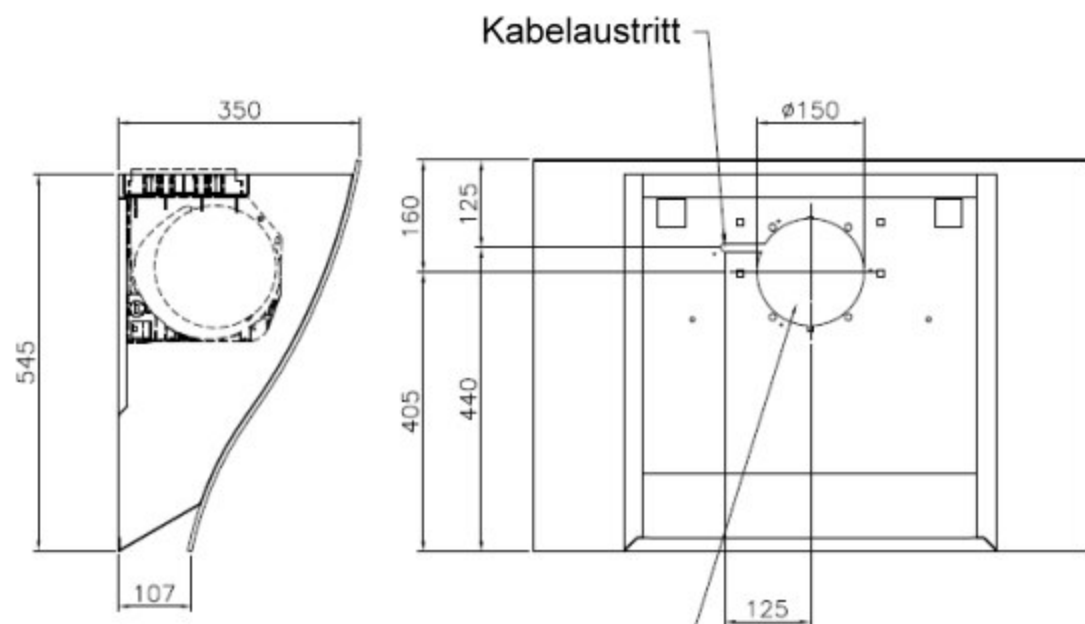
Rückansicht mit gedrehtem Motor
